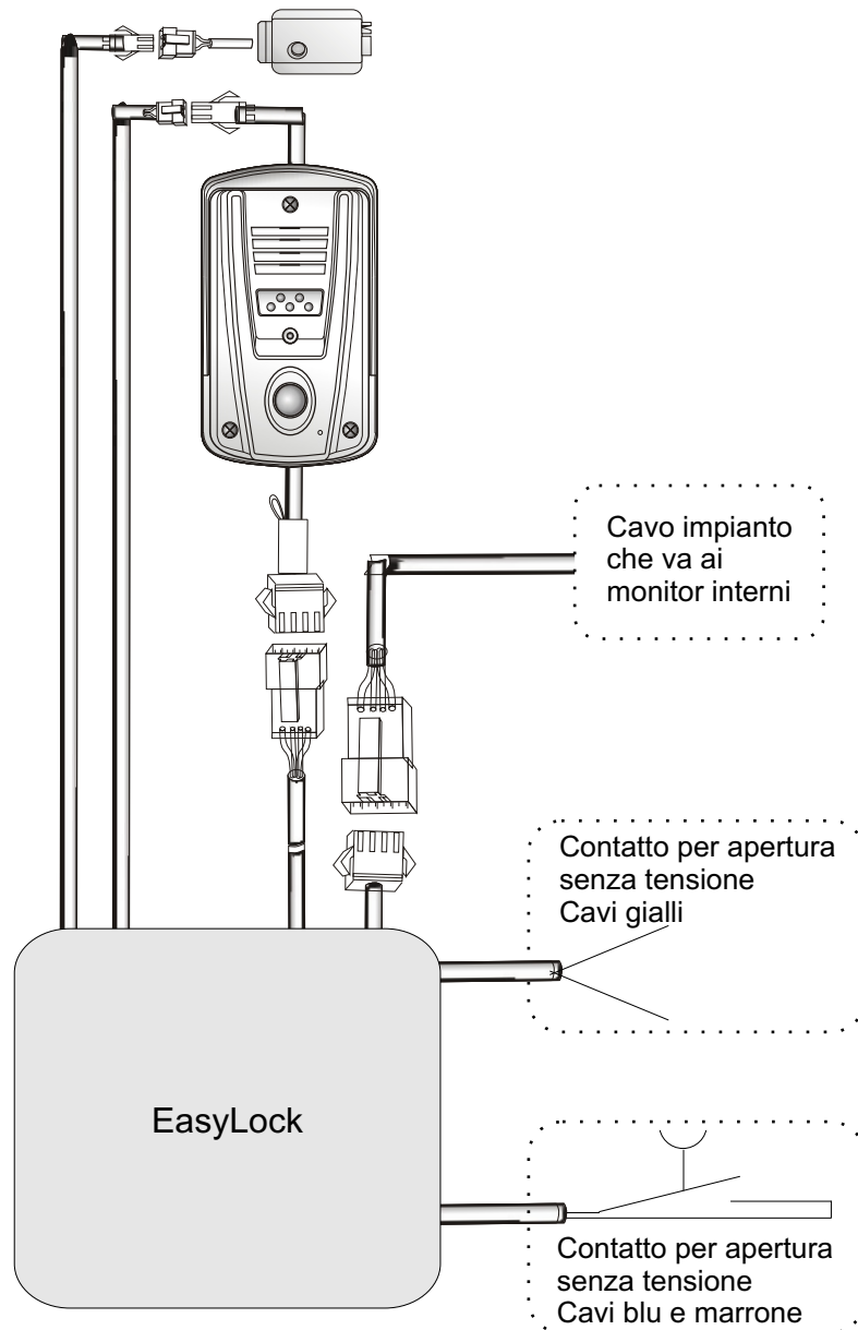
Schema di collegamento con Easy 100
